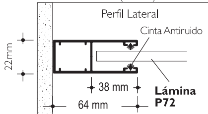
Corte Perfil Lateral (Detalle)
