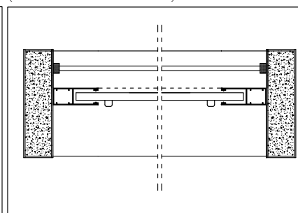
DENTRO DE VANO (PERFIL NO EMPOTRADO)
