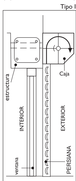
Fuera de vano (superficie de la ventana libre)
