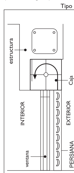
Dentro de vano (ventana integrada)
