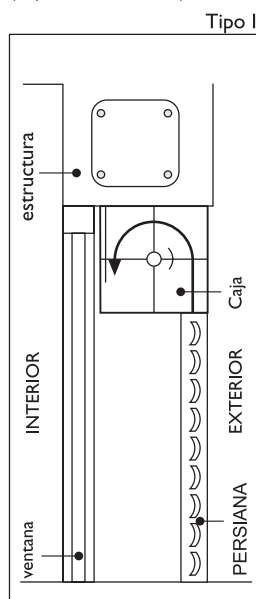
* Dentro de vano Dentro de vano (deja cámara de aire)
