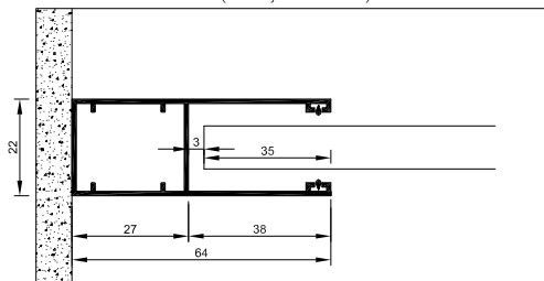
Corte Perfil Lateral (Dibujo Técnico)
